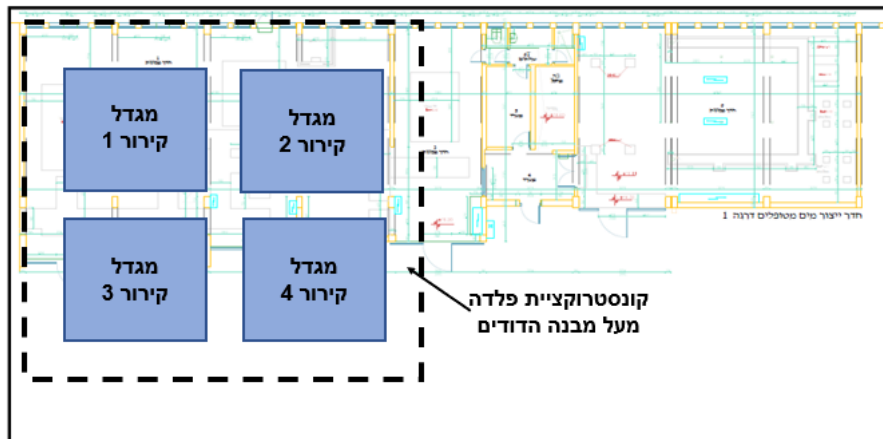
איור 8 – דוגמה עקרונית לפריסת מגדלי קירור על קונסטרוקציית הפלדה מעל מבנה הדודים
