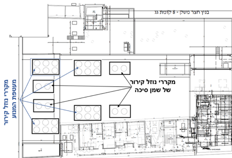
איור 9 – דוגמה עקרונית לפריסת מגדלי קירור על קונסטרוקציית הפלדה מעל מבנה הדודים
