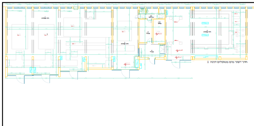
איור 7 – תוכנית מבנה הדודים והחצר לפניו
