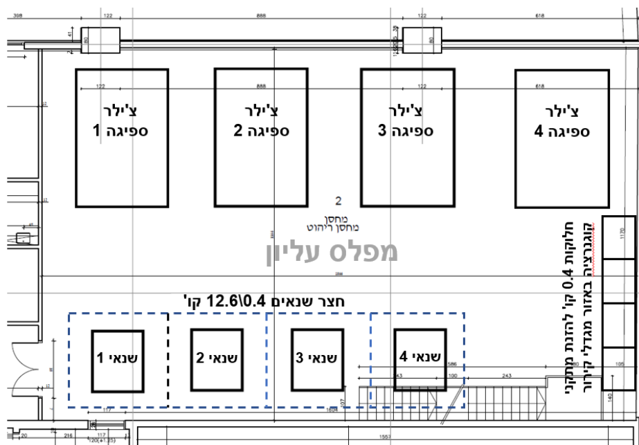
איור 6 - דוגמה עקרונית לפריסה של מתקנים במפלס העליון של חלל הקוגנרציה
